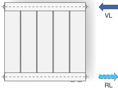
Reitender Anschluss
