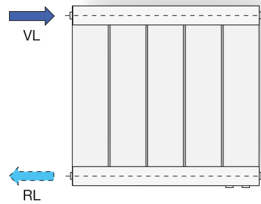
Reitender Anschluss
