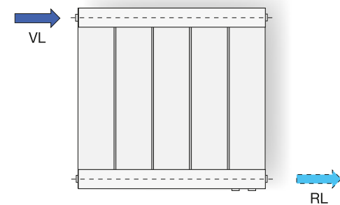
Wechelseitiger Anschluss
